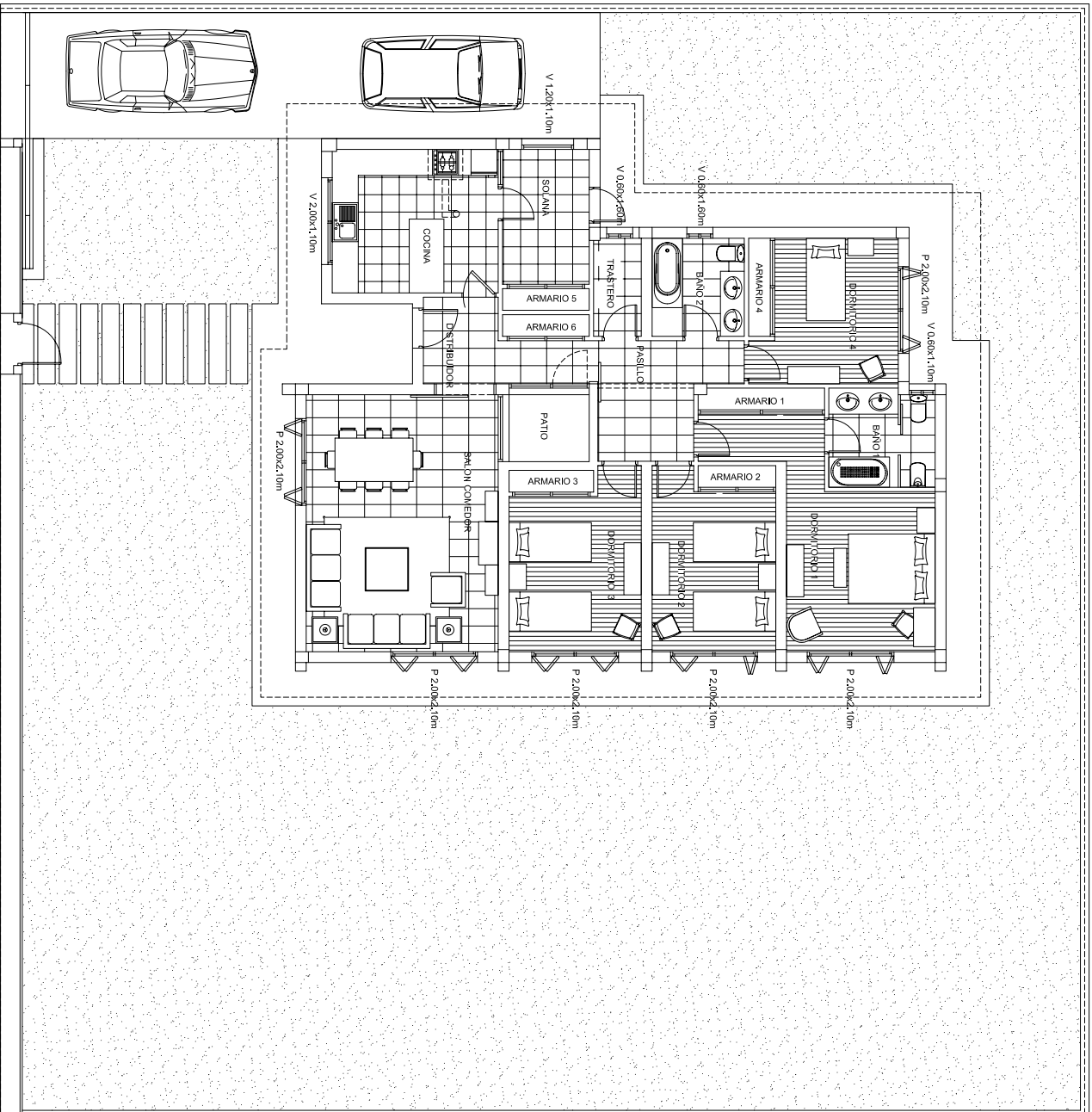
Planta de vivienda
